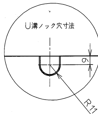
ノック穴詳細図
